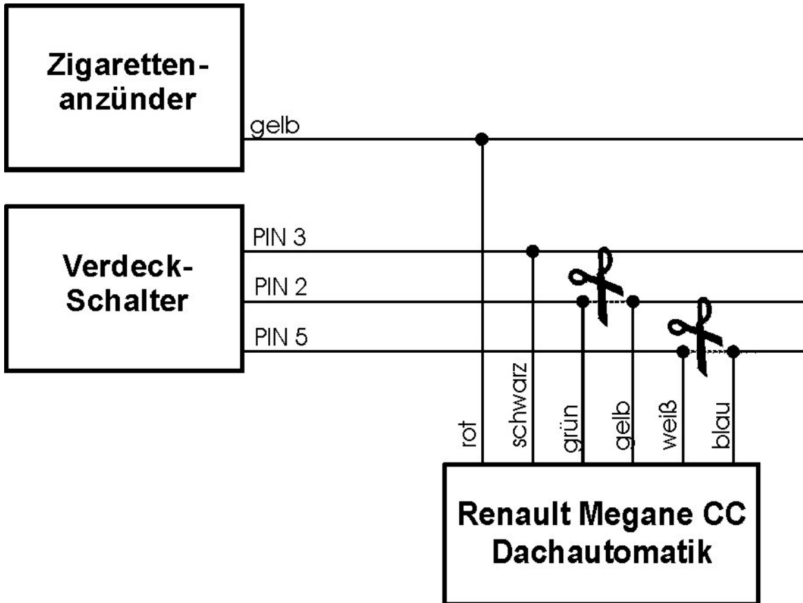
Bild 7: Verkabelung des Dachautomatikmoduls
